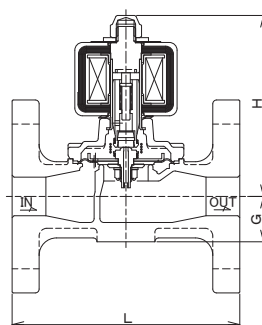
WF-22,22N型
