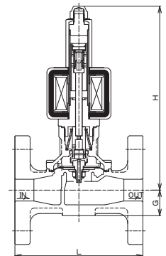
WF-22C,22CN型
