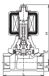
PS-22型
