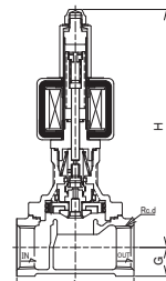
PS-22C型
