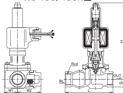
WS-43C, 43CN型
