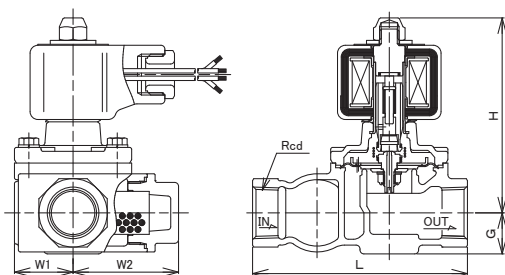
WS-43, 43N型
