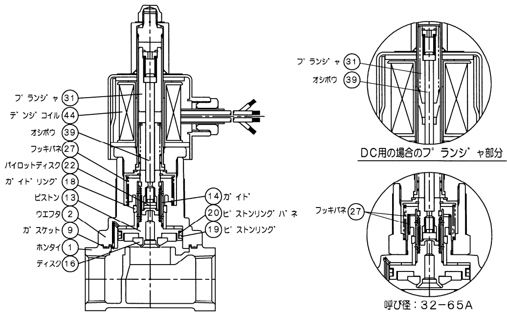
PS-13C型【ホンタイ ① ストレーナ部】 (キャップを外した状態)
