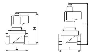
※5.面間寸法は旧PS-15,15C型と同じです。
