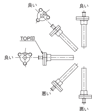
図3. 感熱筒取付け方向
