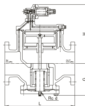
呼び径100~200
