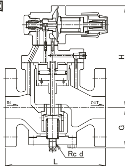
呼び径15~80
