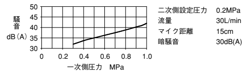
一次側圧力変化時の騒音特性
