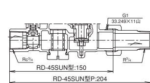
RD-45SUN型P(出口オスユニオン継手)
