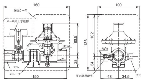
RD-45SN型(入口・出口共Rcねじ)
