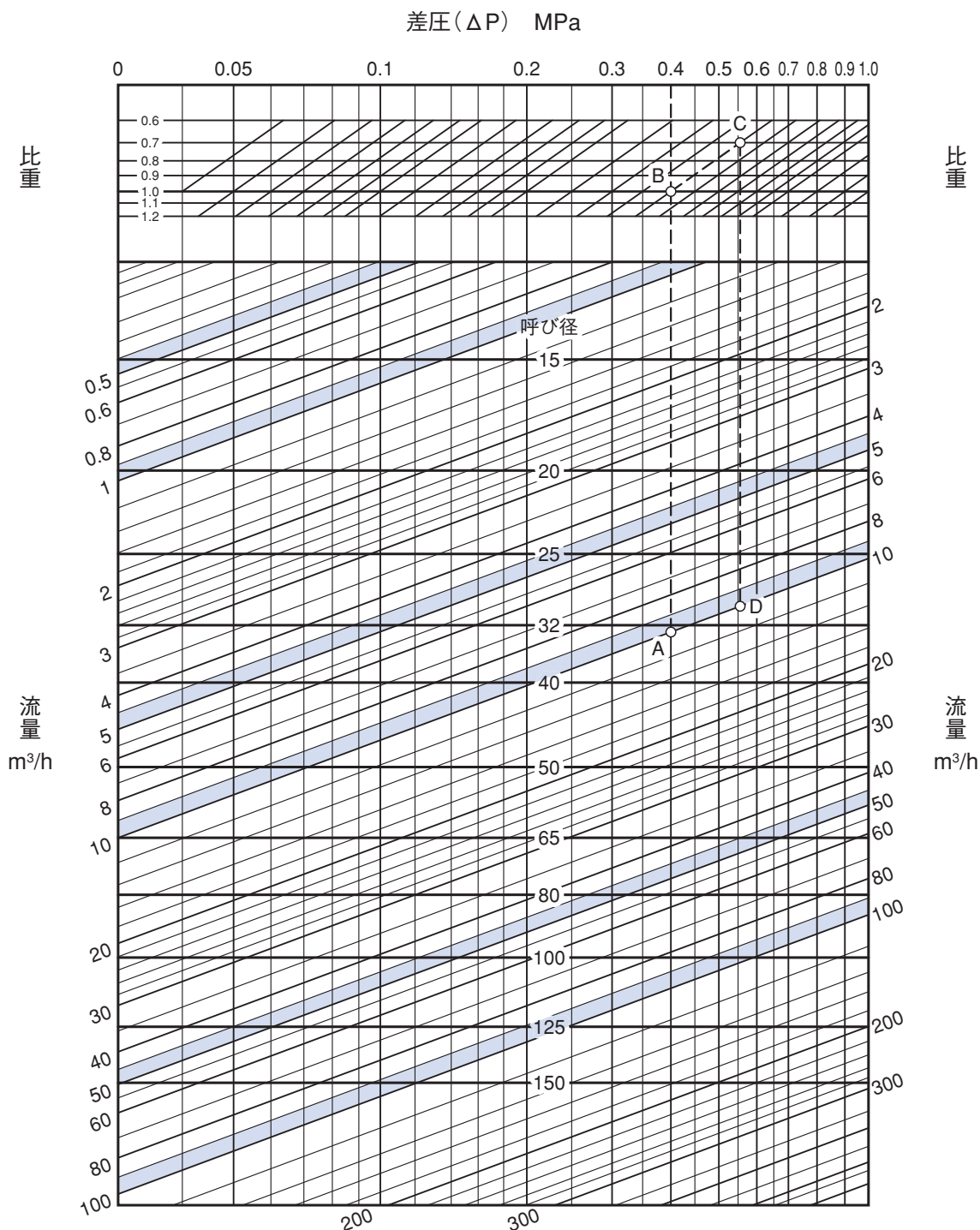
呼び径選定図表〈液体用〉
