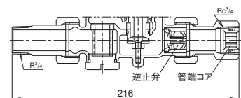
オス・メスユニオン継手の場合
