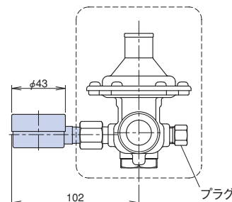
圧力計A型の場合
