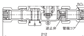
メスユニオン継手の場合
