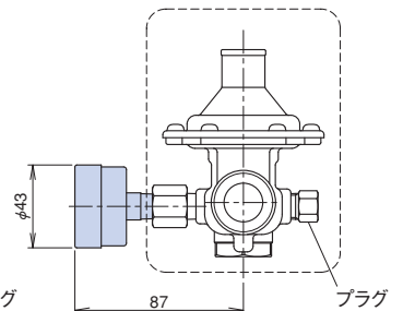
圧力計D型の場合
