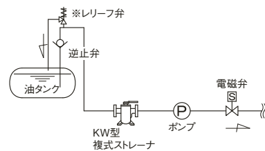
図5. レリーフ弁取付例略図
