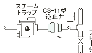
図2. トラップ出口側水抜きの例
